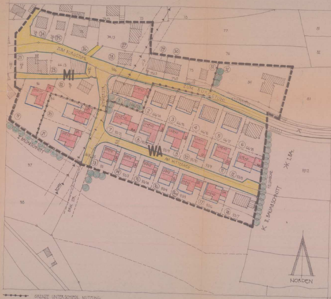
BEBAUUNGSPLAN PIRK - ZUM BURGSTUHL LAGEPLAN M 1/1000
